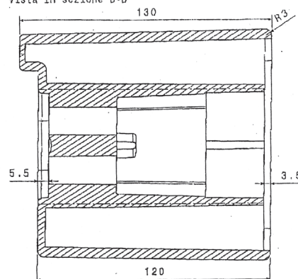
Vista in sezione B-B
